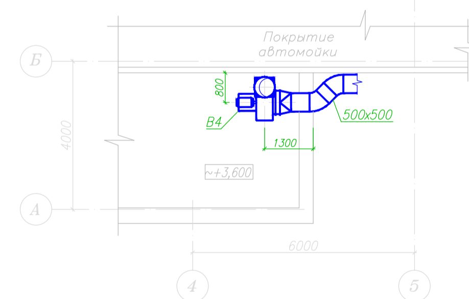
Фрагмент плана на отм. +3,600
